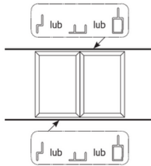
Zweiflügeliges einspuriges Insektenschutz
