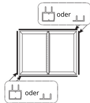
Zweiflügeliges zweispuriges Insektenschutz mit Rahmen
